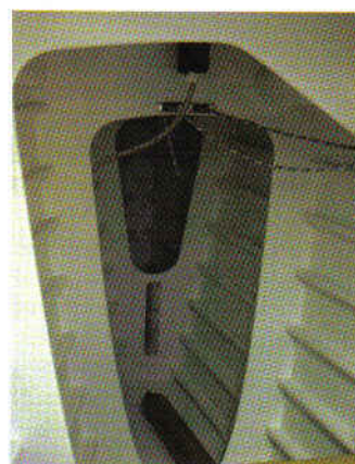
Das aufwändige Innenskelett der Abraxas 10.50 CR.
