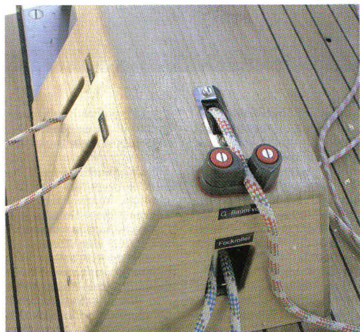
Zentrale Trimmeinheit im Cockpit.
