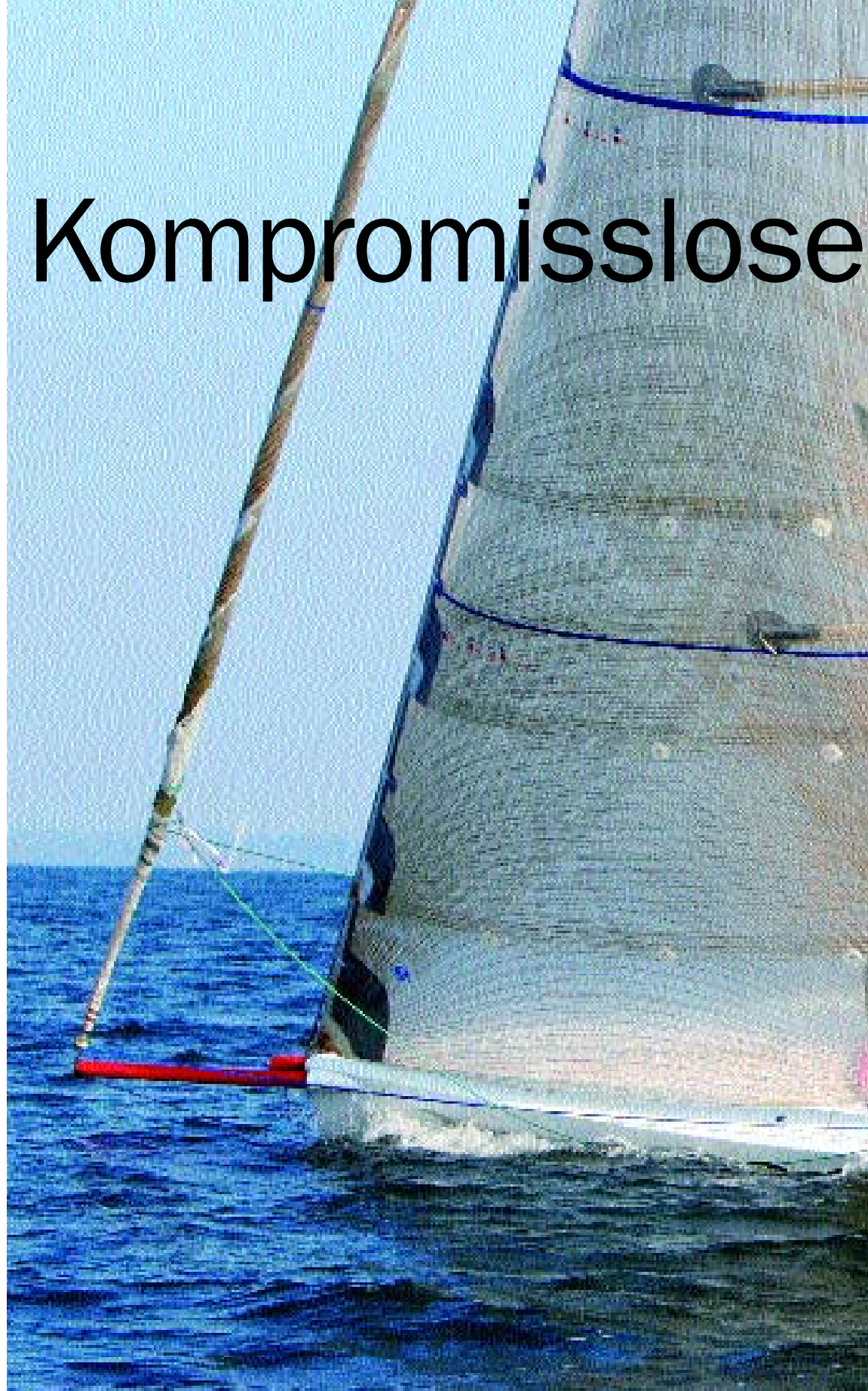
Gewaltige Segelfläche: 86 Quadratmeter Tuch hängen am 16 Meter hohen Carbon Mast, und das bei einer Bootsbreite von 3,50 Metern auf der Deckskante platziert werden kann und dort ein hohes aufrichtendes Moment liefert.
